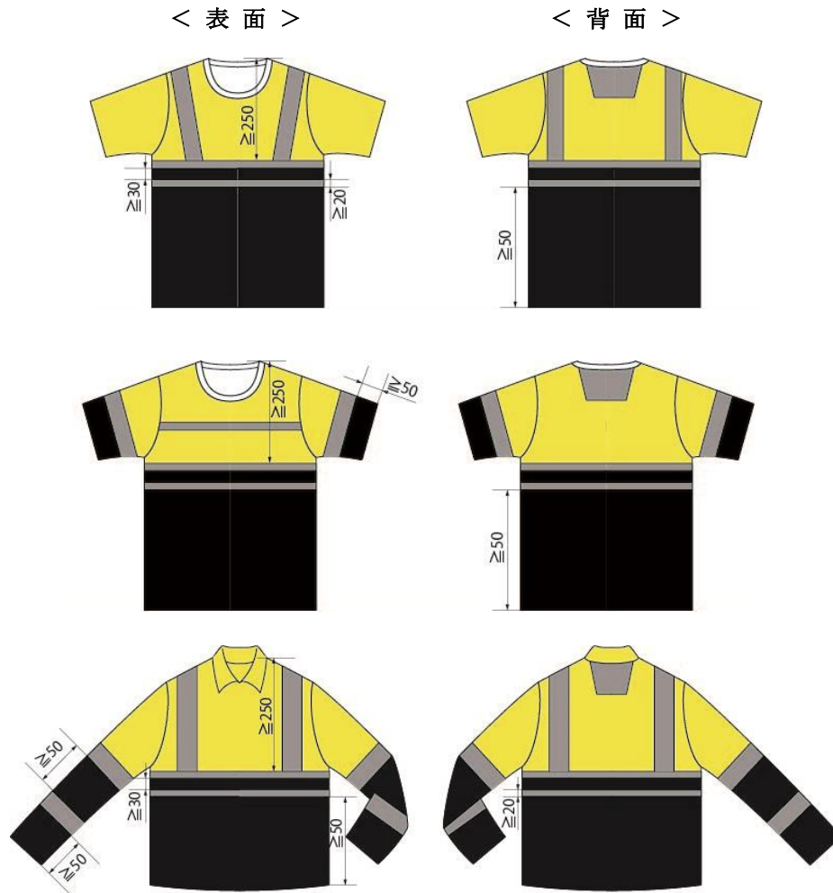
図 2—胴部と腕部を覆う自転車通学者用高視認性安全服の例
